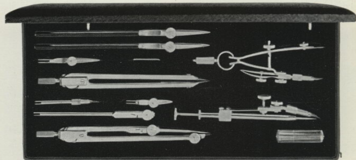
C 31 2/3003 Handreißfedern 3073 Fallnullenzirkel mit Blei- und Federeinsatz 3086 Federzirkel mit Blei- und Federteil 3113 Stechzirkel 3147 Einsatzzirkel mit Nadel-, Blei-, Federeinsatz und Verlängerungsstange 3177 Büchse mit Nadel und Minen 3178 Schraubenschlüssel
