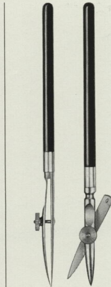
1003 normale Handreißfeder
