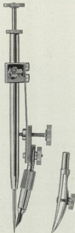
3073 Fallnullenzirkel mit Blei- und Federeinsatz
