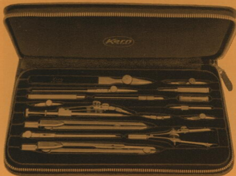
RA 330 1003 Handreißfeder 1043 Starkstrichfeder 1061 Pikiernadel 1073 Fallnullenzirkel mit Blei- und Federeinsatz 1087 Federzirkel mit Nadel-, Blei-, Federeinsatz 1113 Stechzirkel 1147 Einsatzzirkel mit Nadel-, Blei-, Federeinsatz und Verlängerungsstange 1171 Einsatzhalter 1176 Zentrumscheibe 1177 Büchse mit Nadeln und Minen 1178 Schraubenzieher Dieses Reißzeug ist auch mit Metalletui A 330 erhältlich
