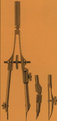
1087 Federzirkel mit Mitteltrieb mit Nadel-, Blei- und Federeinsatz. Holzetui E 1087 extra
