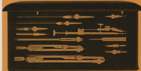
B 123 2001 Handreißfeder 2003 Handreißfeder 2073 Fallnullenzirkel mit Blei- und Federeinsatz 2133 Einsatzzirkel mit Nadel-, Blei-, Federeinsatz 2147 Einsatzzirkel mit Nadel-, Blei-, Federeinsatz und Verlängerungsstange 2179 Schraubenzieher mit Nadeln und Minen
