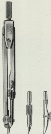
1133 Kleiner Einsatzzirkel mit Nadel-, Blei- und Federeinsatz
