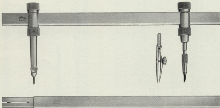
1100 Metallstangen­zirkel mit Feineinstellung, bestehend aus Grundstange 23 cm, Verlängerungsstange 20 cm, Spitzenteil und Einsatzteil mit Blei- und Federeinsatz
