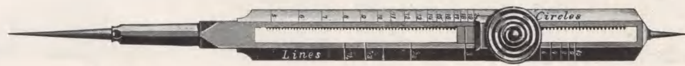
Nr. 26. Reduktionszirkel, 18,5 cm, mit Mikrometertrieb, Linien- und Kreisteilung.
