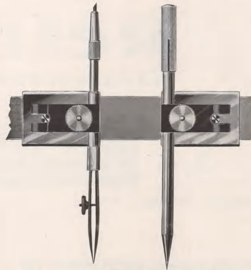
Nr. 25. Stangenzirkel mit Reißfeder, Bleieinsatz und Zentrierspitze.
