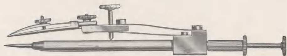
Nr. 6. Fallnullenzirkel.
