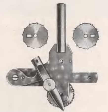
Nr. 30. Kreis-Punktierapparat.
